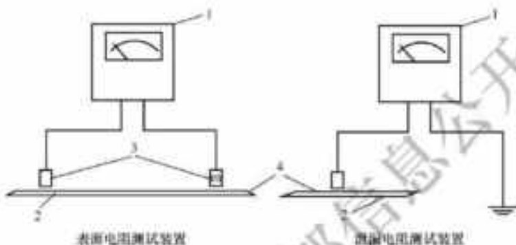
图 C.15.2 表面静电性能测试装置
